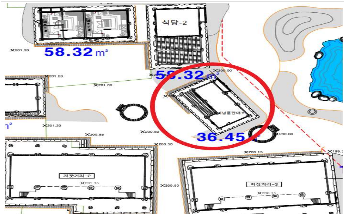
한국문화테마파크 기념품판매소 현장 도면
